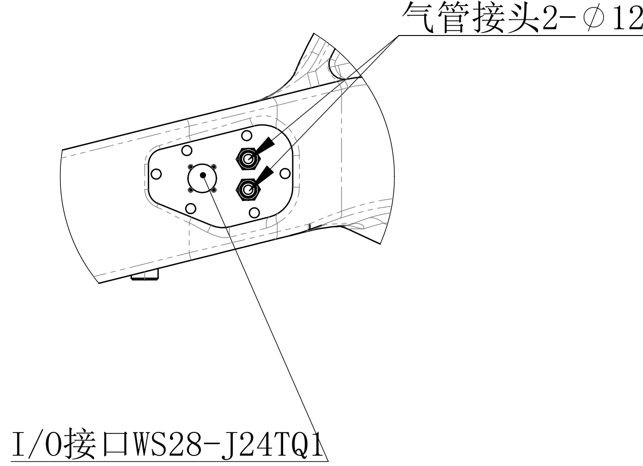
视图I
