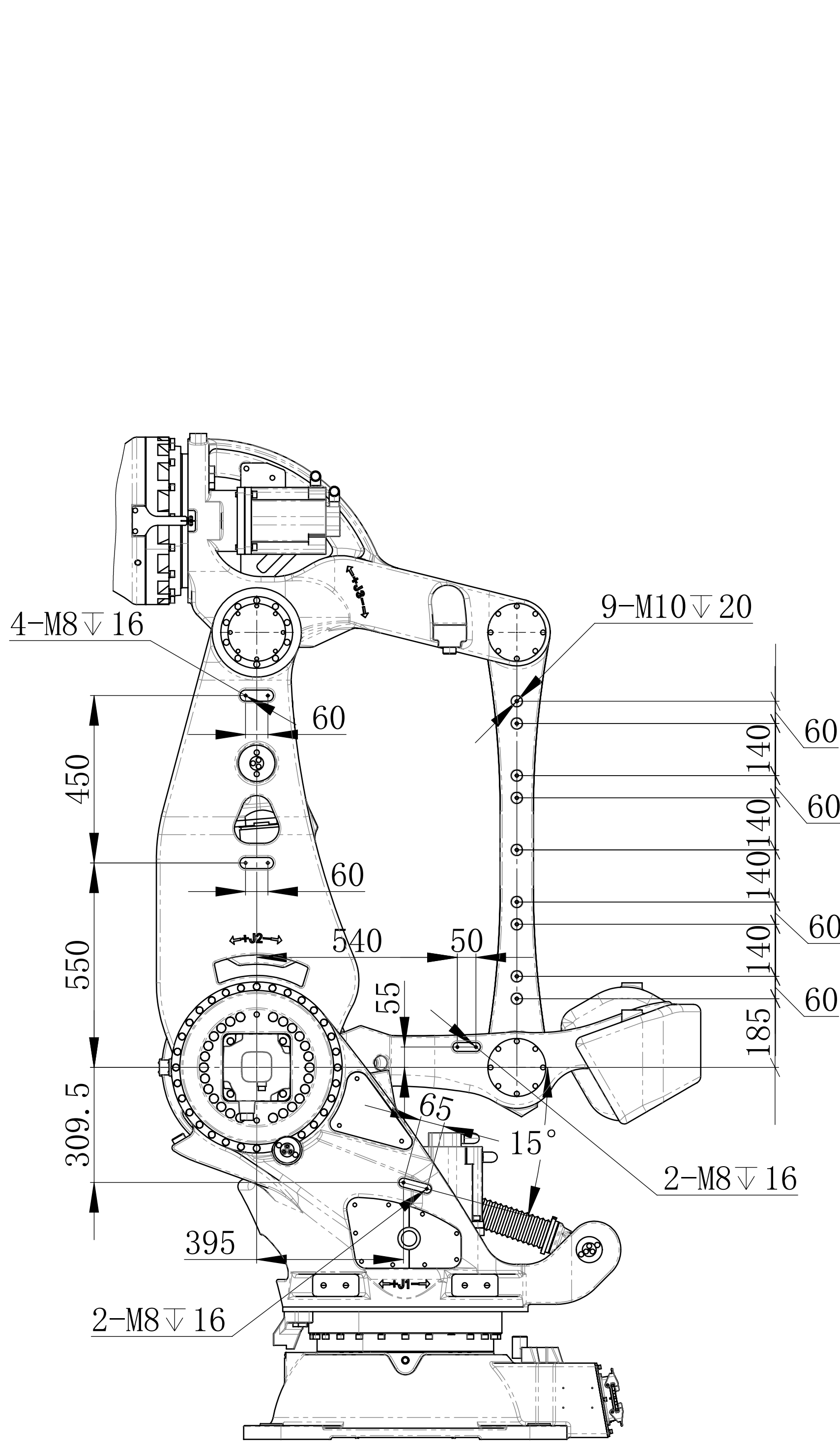
设备面安装尺寸
