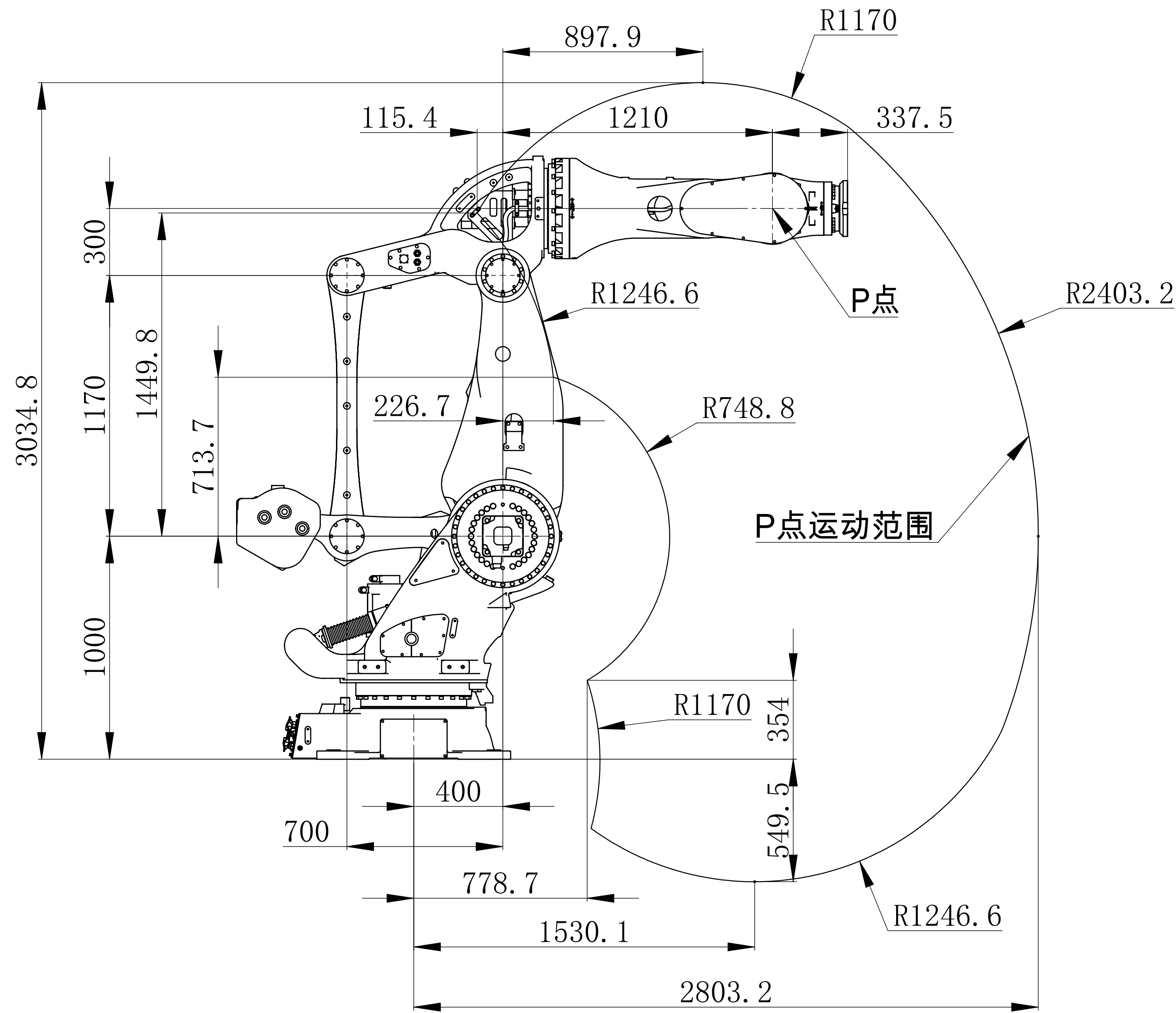
动作范围图
