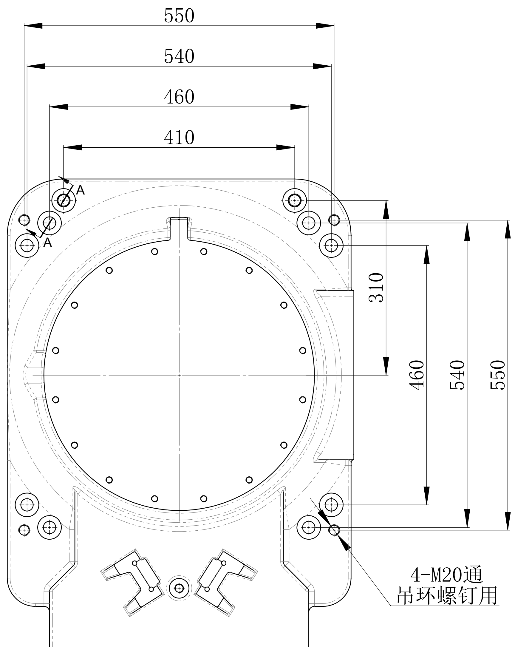
底座安装接口
