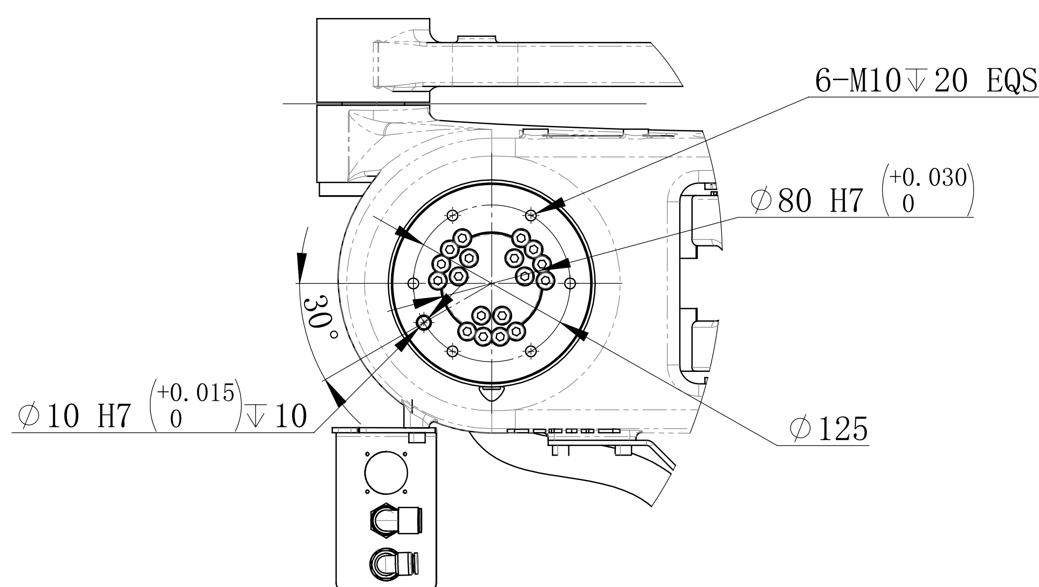
底座安装接口 视图比例1:5
