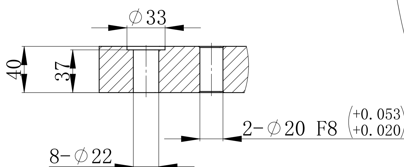
\frac{A-A}{1:2}
