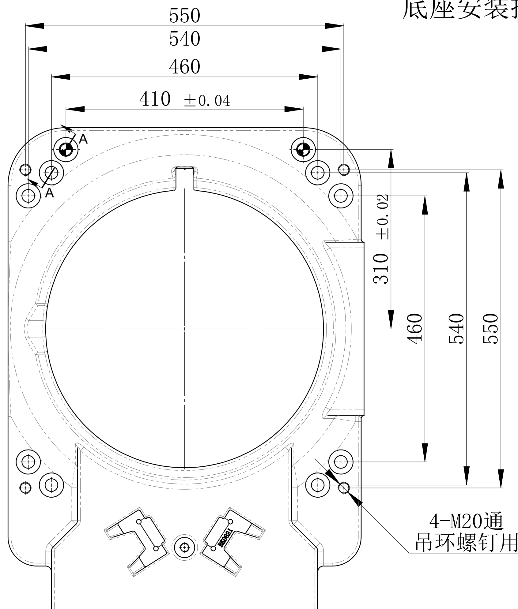
底座安装接口
