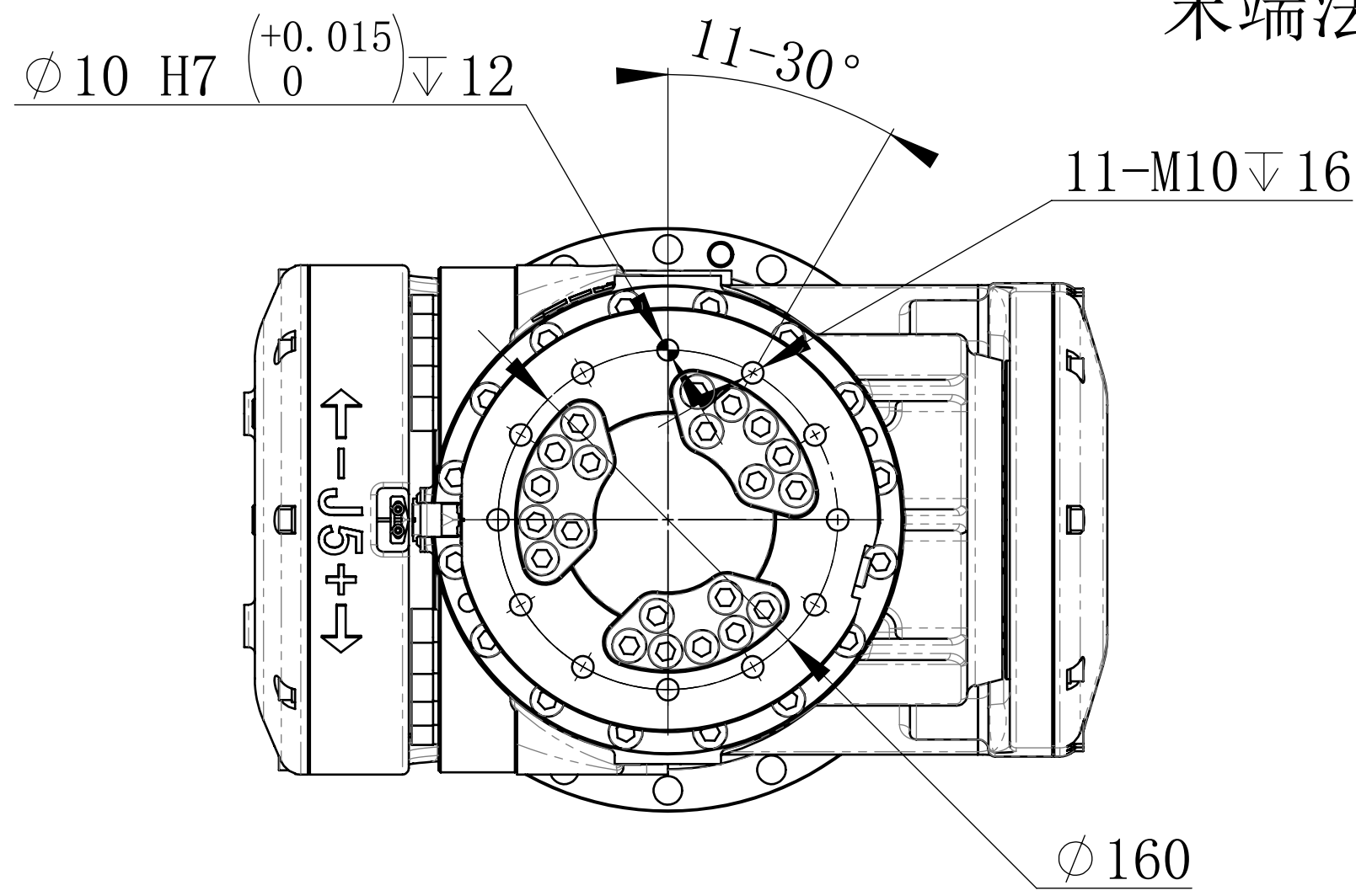
末端法兰安装接口
