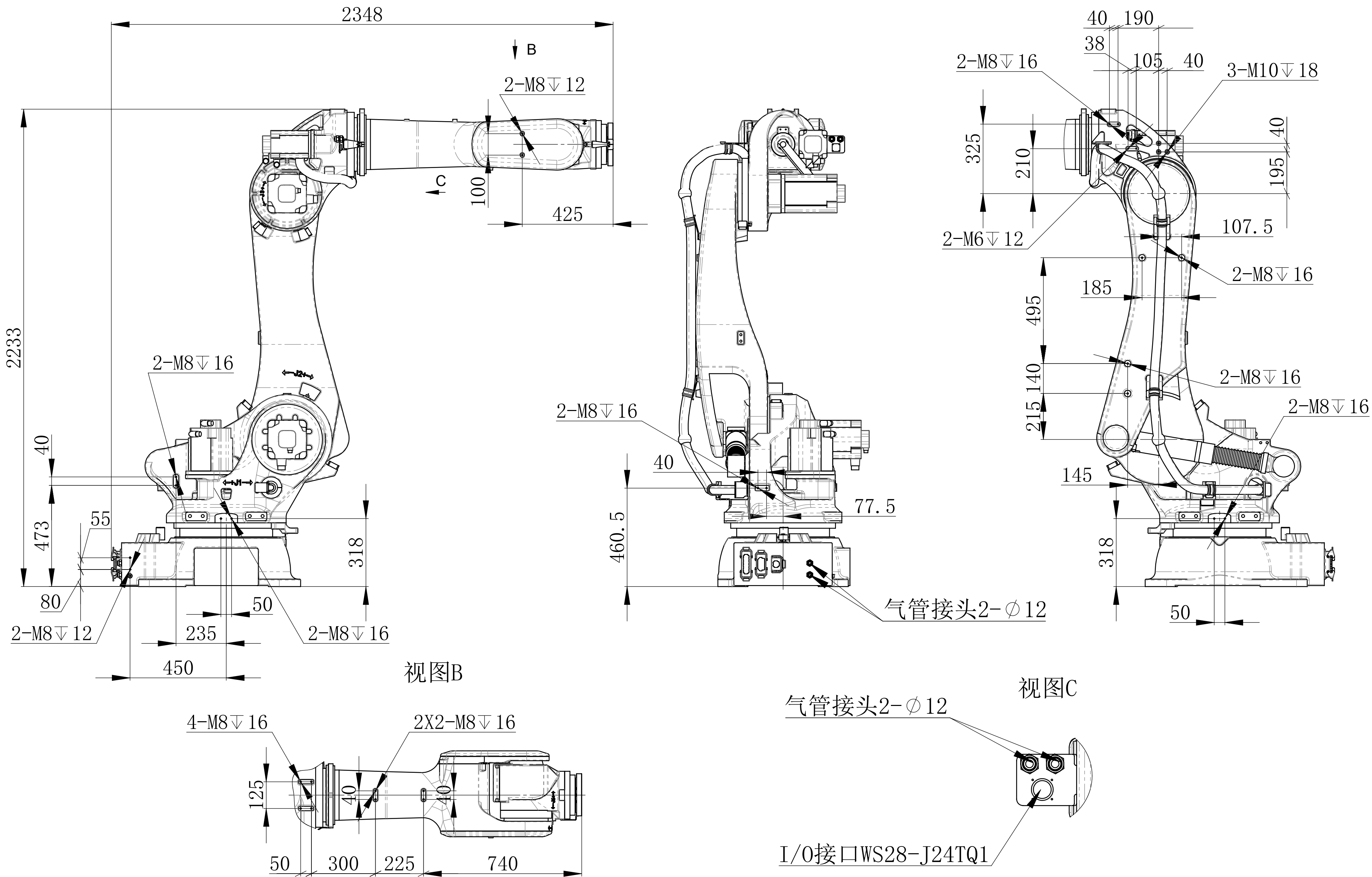
设备面安装尺寸
