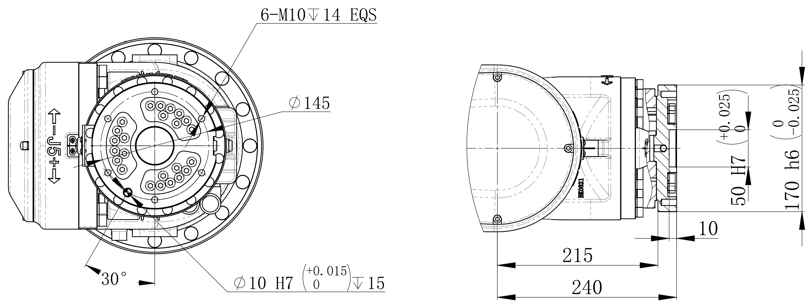
末端法兰安装接口
