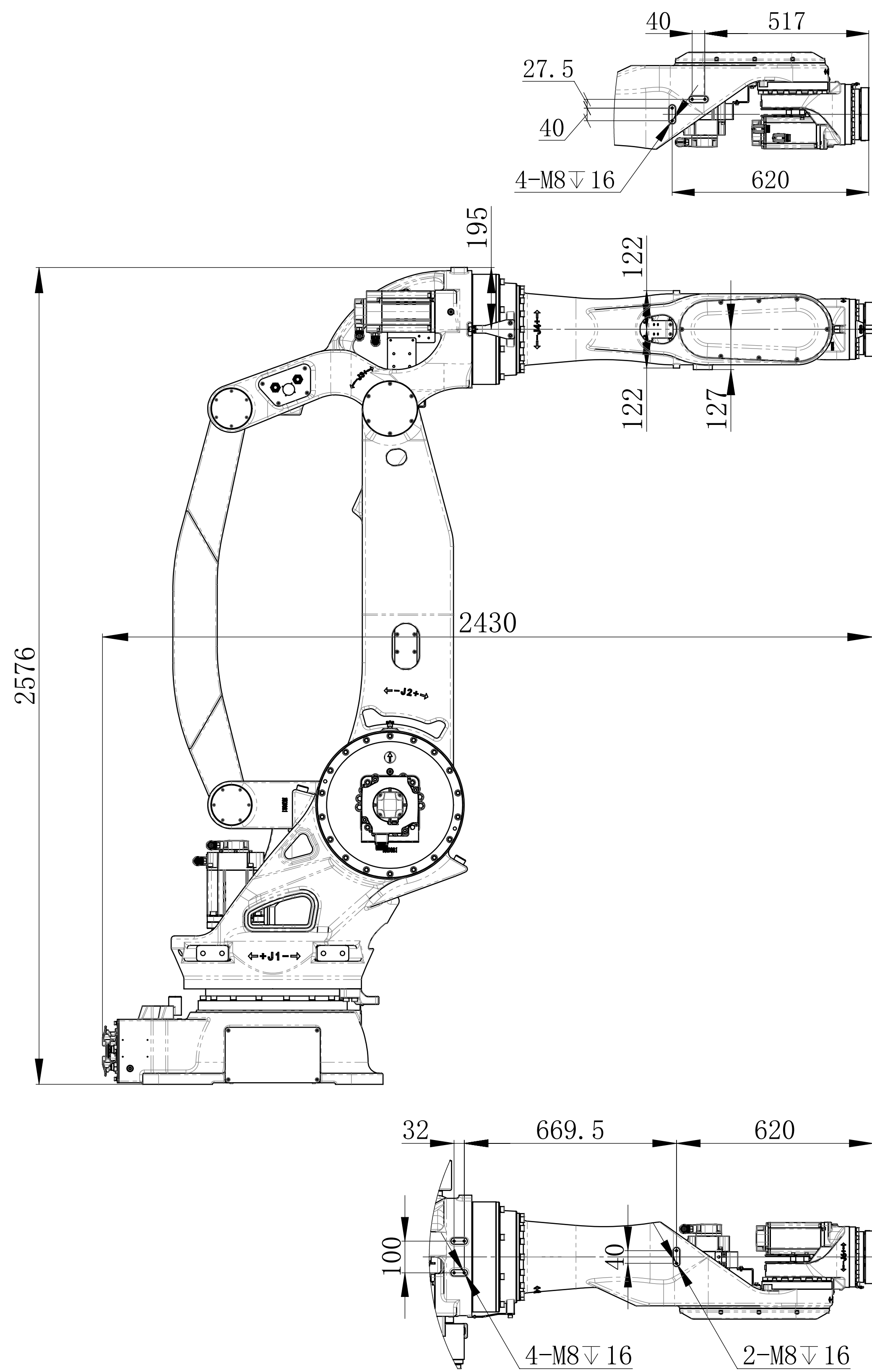
底座安装接口
