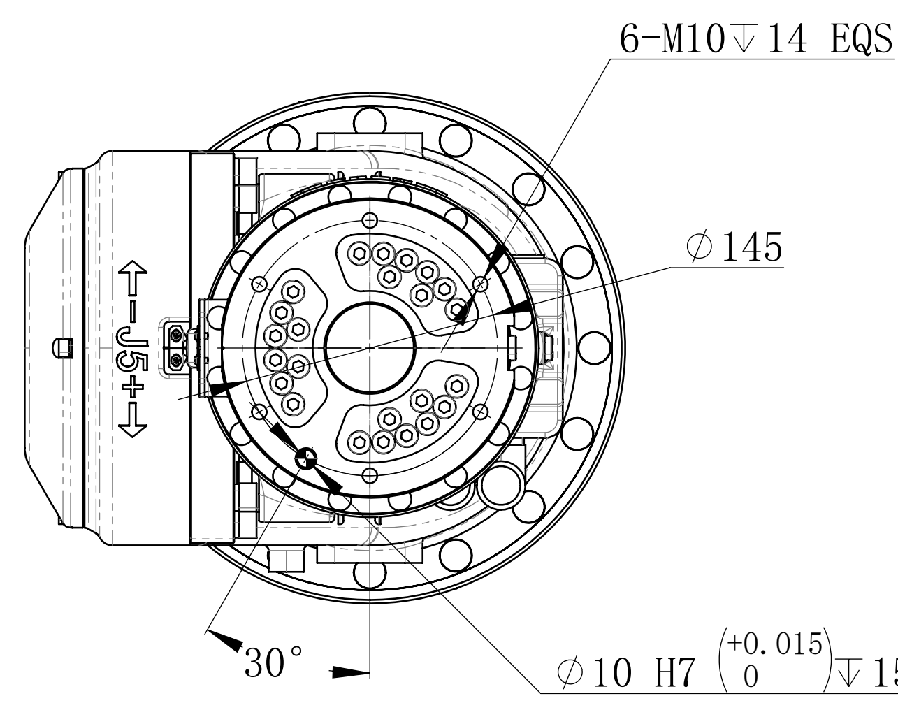
末端法兰安装接口
