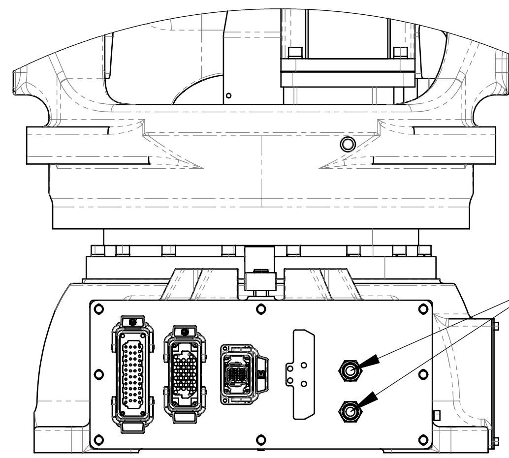
气管接头2- \phi 12
